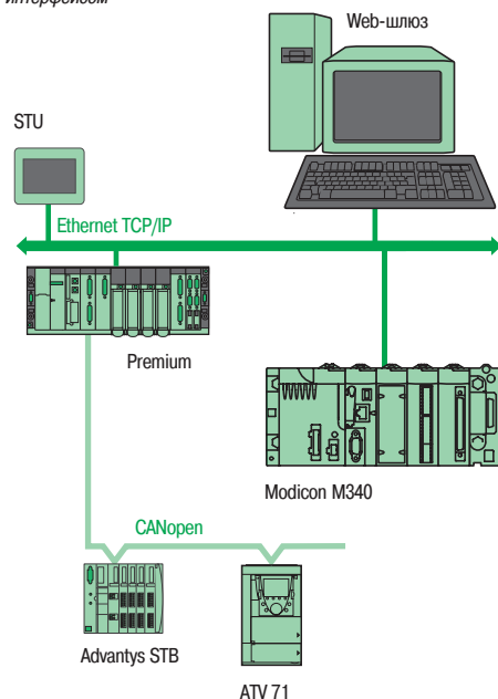
Пример архитектуры на базе сети Ethernet TCP/IP
